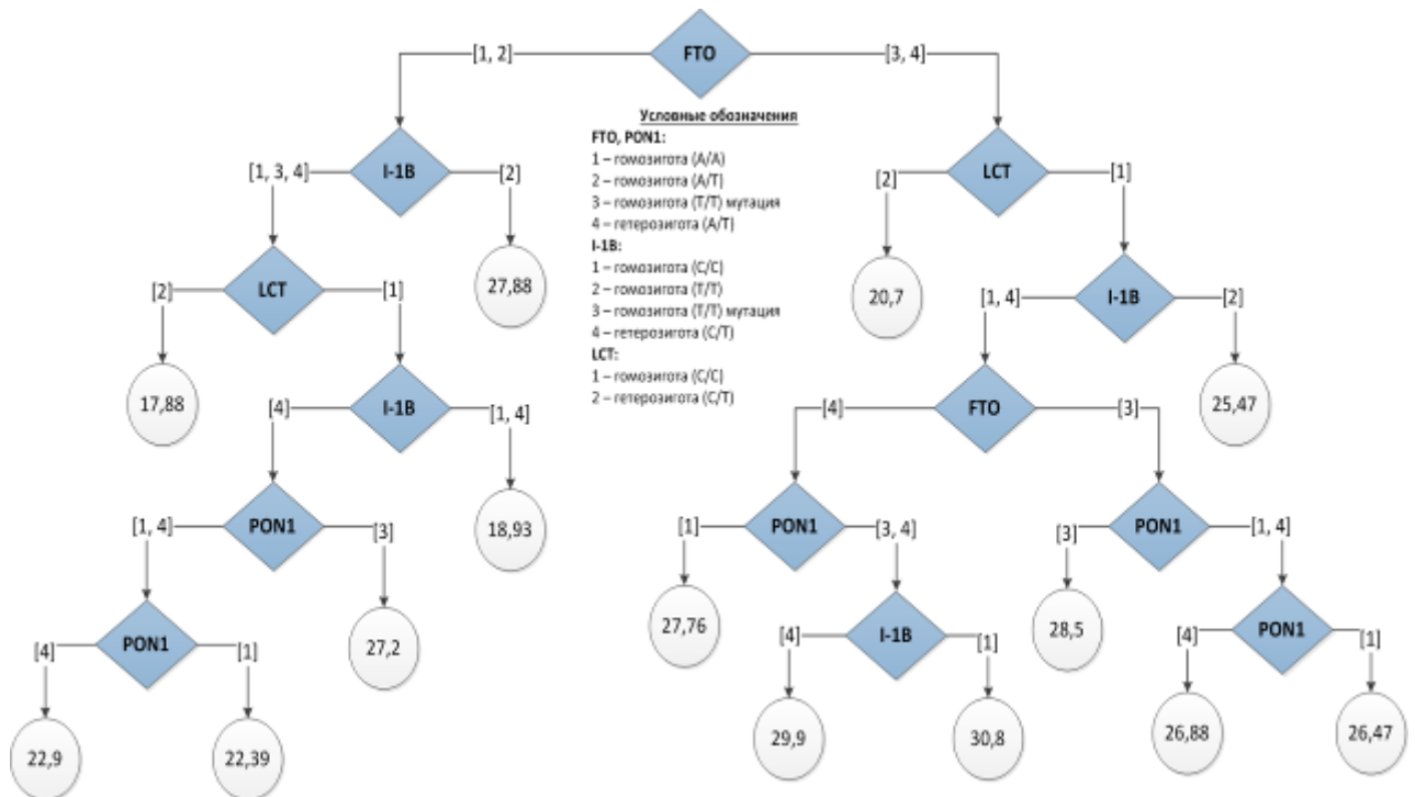
Рис. 3.20. Дерево рішень
